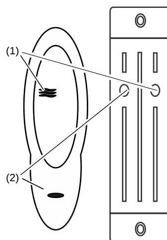
Afbeelding 4: ATS1190/ATS1192-lezers
