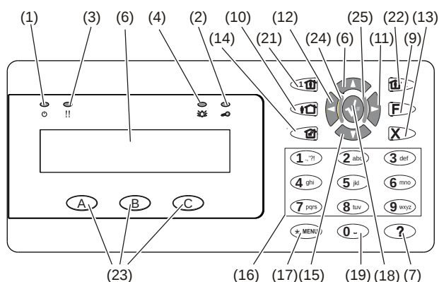
Figuur 2: ATS113x-gebruikersinterface
